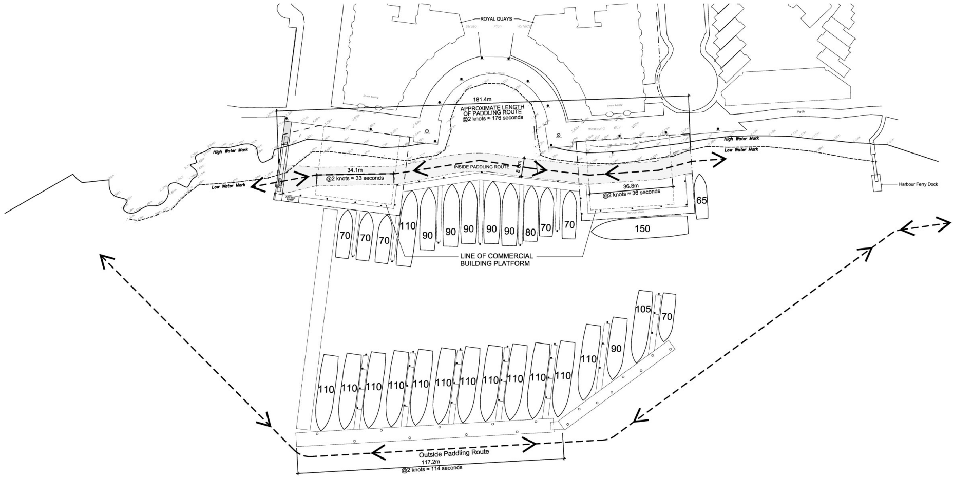
1 SITE PLAN A.1.0
